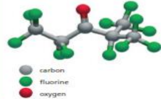
Novec™ 1230 molecule
