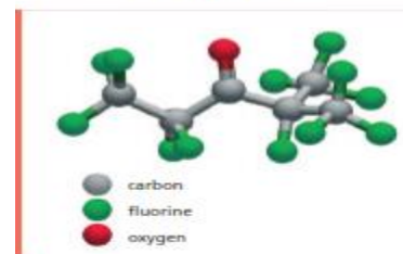
Novec™ 1230 molecule
